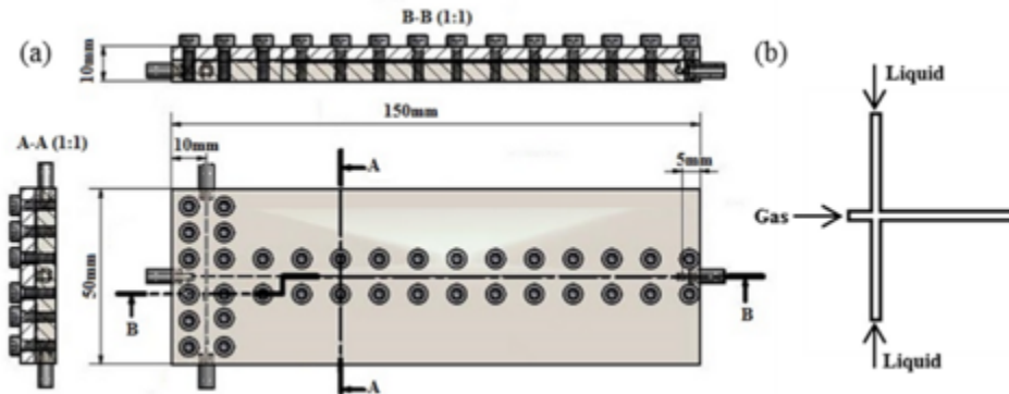
Figure 43. Schéma du microcanal utilisé pour l'étude de la contribution du transfert de matière lors de la formation de bulles, extrait de (Yang et al., 2016). Canaux de section carrées de 500 µm.
