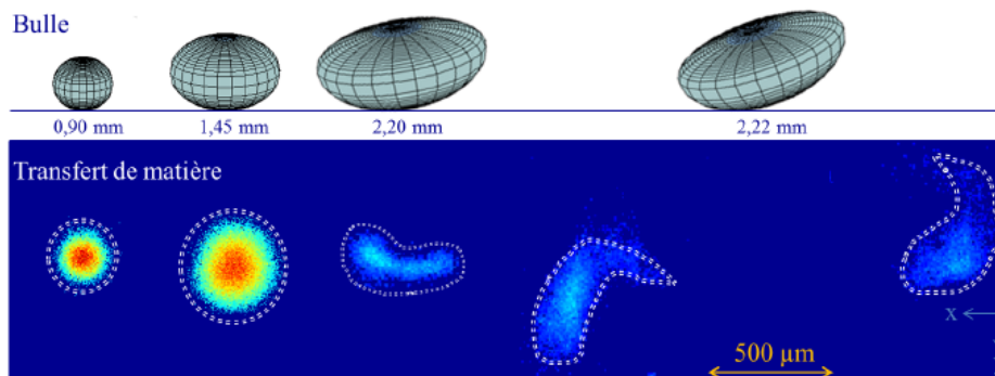
Figure 77. Impact du diamètre équivalent d'une bulle d'air sur le transfert de matière visualisé.
