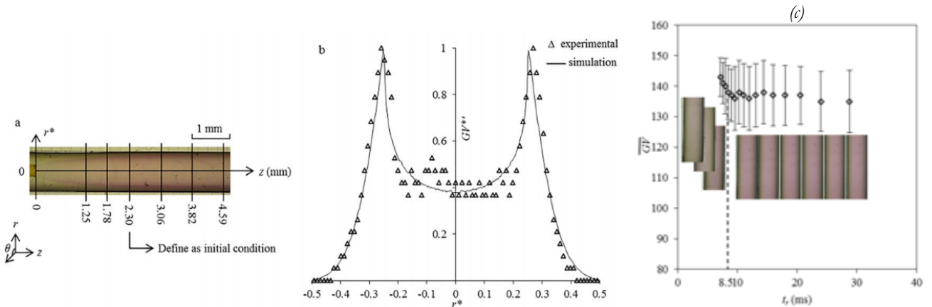
Figure 32. (a) Mesure du coefficient de diffusion par un dispositif microfluidique expérimental, extrait de (Yang et al., 2017) (b) Comparaison des profils expérimentaux et théoriques pour la mesure du coefficient de diffusion de l'oxygène, extrait de (Yang et al., 2017) (c). Mesure du temps de réaction de la réaction colorimétrique par analyse à la sortie du micro-mélangeur.
