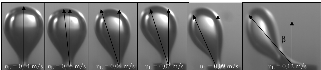
Figure 37. Evolution de la forme et la position de la bulle en fonction de la vitesse de l'écoulement orthogonal.
