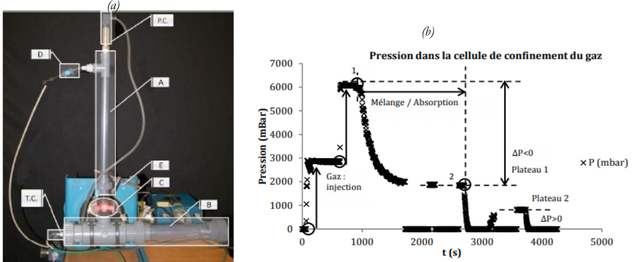
Figure 71. (a) Photographie du montage expérimental. (b) Illustration d'une manipulation grâce à la pression dans la cellule de gaz.
