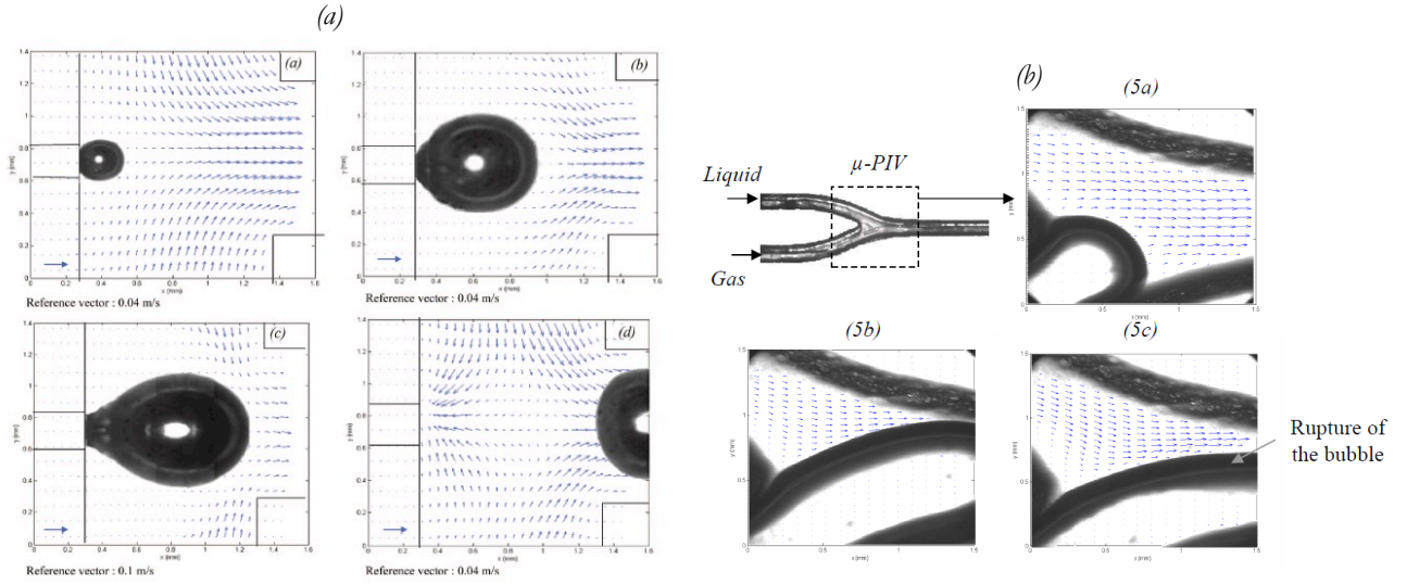
Figure 40. (a) Mesure du champ de vitesse obtenue par le système \mu -PIV pour la formation d'une bulle de 10^{-9} \text{ m}^3 dans un micro-système de type « flow focusing » (d'angle de 180^\circ ). (b) Mesure du champ de vitesse obtenue par le système \mu -PIV pour la formation d'une bulle de 1,4 \cdot 10^{-9} \text{ m}^3 dans un micro-système de type « T » d'angle 60^\circ de section circulaire de 800 \mu\text{m} .
