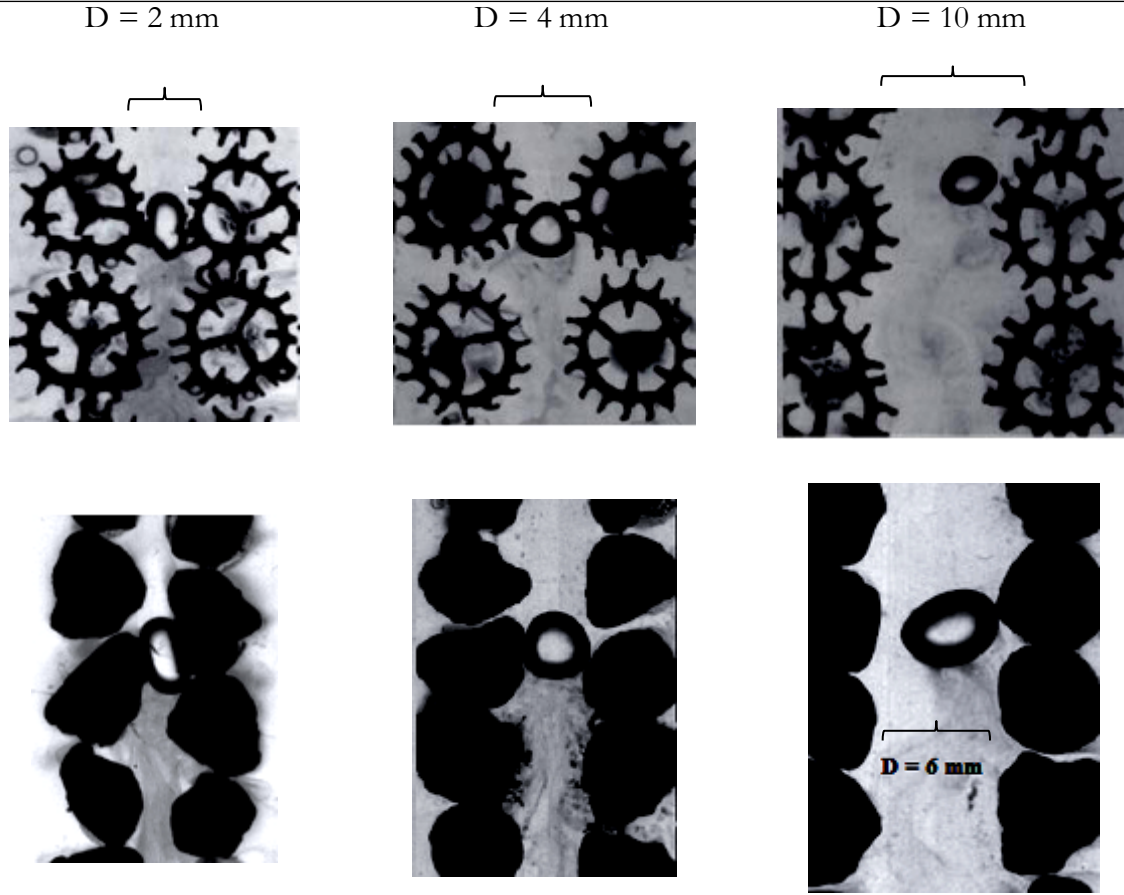
Figure 54. Visualisation du transfert de matière par colorimétrie autour d'une bulle en ascension dans le Météor (en haut) et Biolite P3.5 (en bas)
