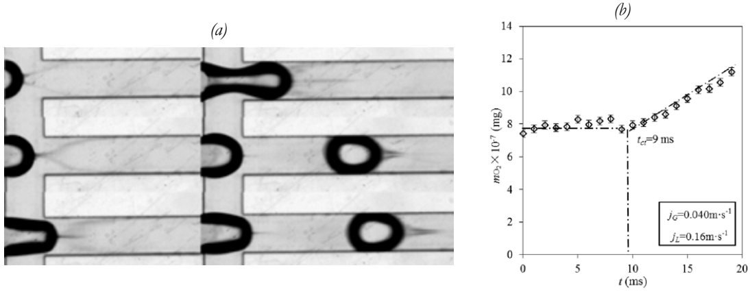
Figure 44. (a) Suivi de la formation d'une bulle dans le système « flow focusing » pour j_G = 0.053 \text{ m.s}^{-1} , j_L = 0.27 \text{ m.s}^{-1} . (b) Evolution de la masse transférée en fonction du temps après la formation d'une bulle.
