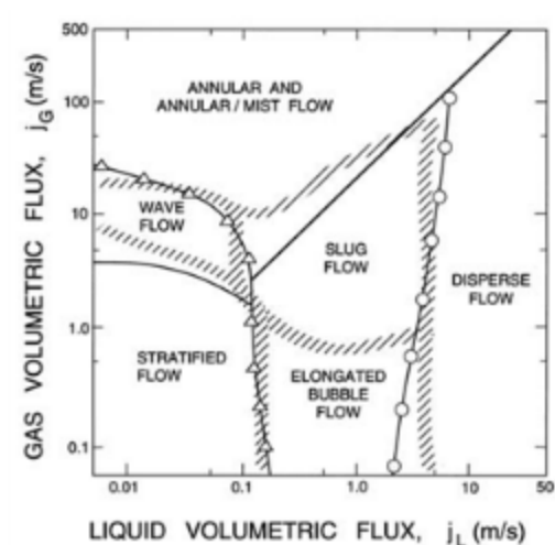
Figure 81. Type de régime d'écoulement gaz-liquide présent en conduite. Extrait de (Abdulmouti, 2014)
