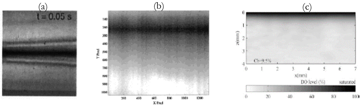
Figure 25. Etude du suivi de la fluorescence au voisinage d'une interface plane. (a) Extrait de Münsterer and Jähne (1998). (b) Extrait de Woodrow and Duke (2001). (c) Extrait de (Herlina and Jirka, 2004).
