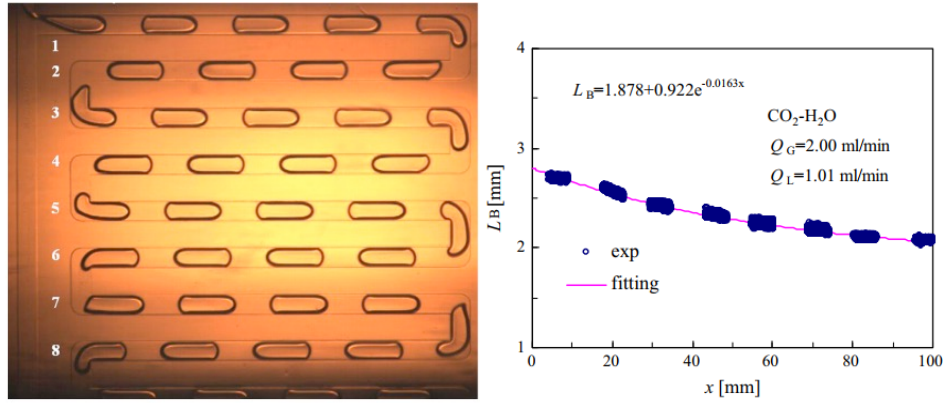
Figure 42. Suivi de la taille de bulles de CO 2 dans un micro-canal par (Yao et al., 2014).
