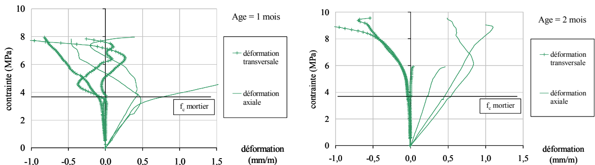
Figure 51- Essais sur sandwiches, comportement des joints de mortier.
