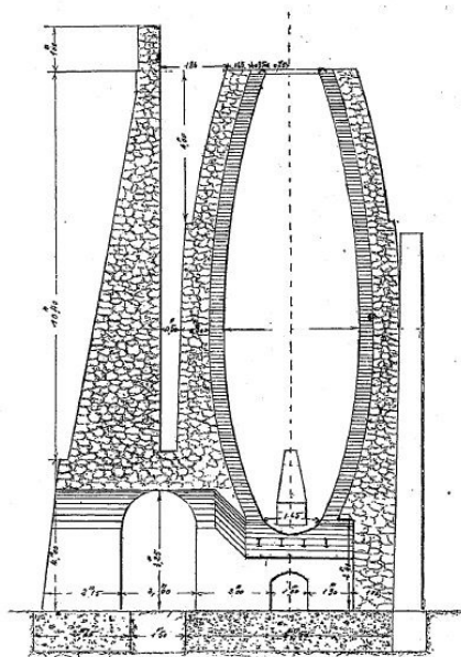
Fig. 2. — Four du Teil.
