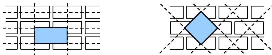
Figure 19 - Cellules de base proposée par A. Cecchi et K. Sab en 2001, pour maçonnerie à joints verticaux continus ou discontinus.
