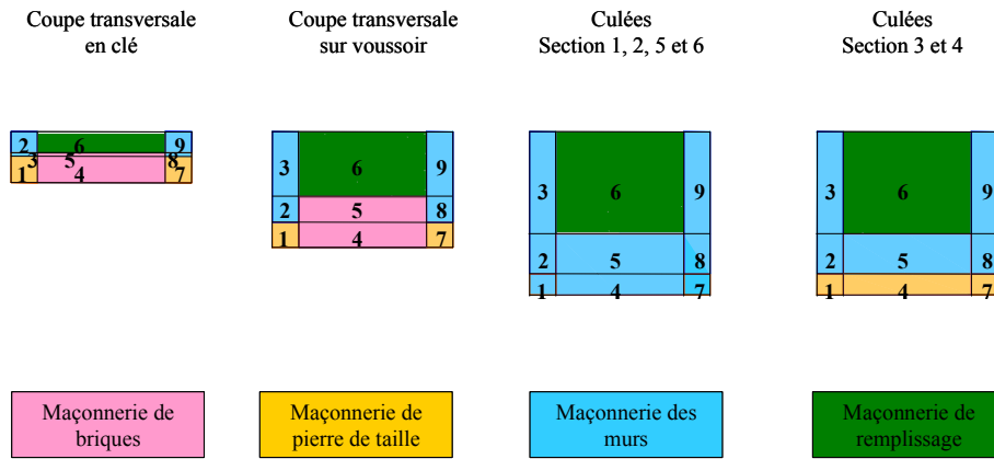
Figure 84 - Modélisation du pont. Position des 4 maçonneries homogénéisées.
