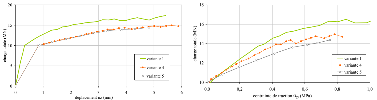
Figure 120 - Comparaison calculs variantes 4 et 5. Déplacement vertical sous essieux et traction transversale.
