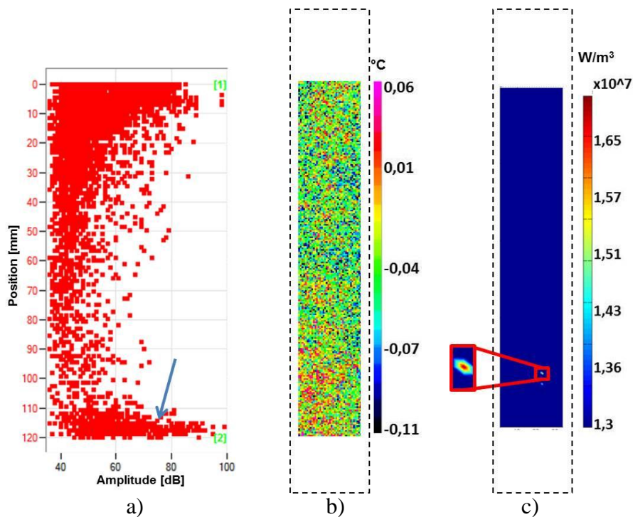
Figure 1. Corrélation spatiale et temporelle d'un évènement acoustique et sa source de chaleur pour un stratifié carbone/époxy sollicité à 0^\circ .
