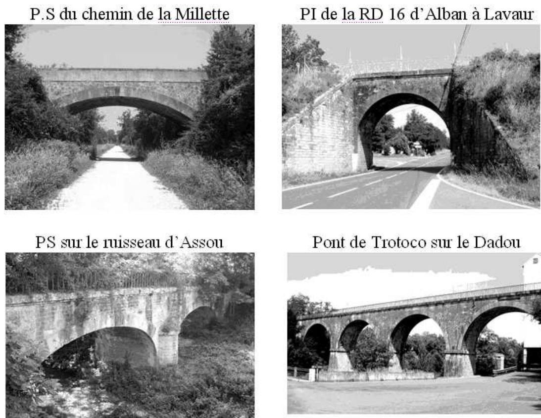
Figure 6. Les principaux ponts en maçonnerie de la ligne : Pont du chemin de la Millette (arc surbaissé), Pont de la RD 16 (plein cintre), Pont sur le ruisseau d'Assou (anse de panier), pont de Trotoco sur le Dadou (plein cintre).
